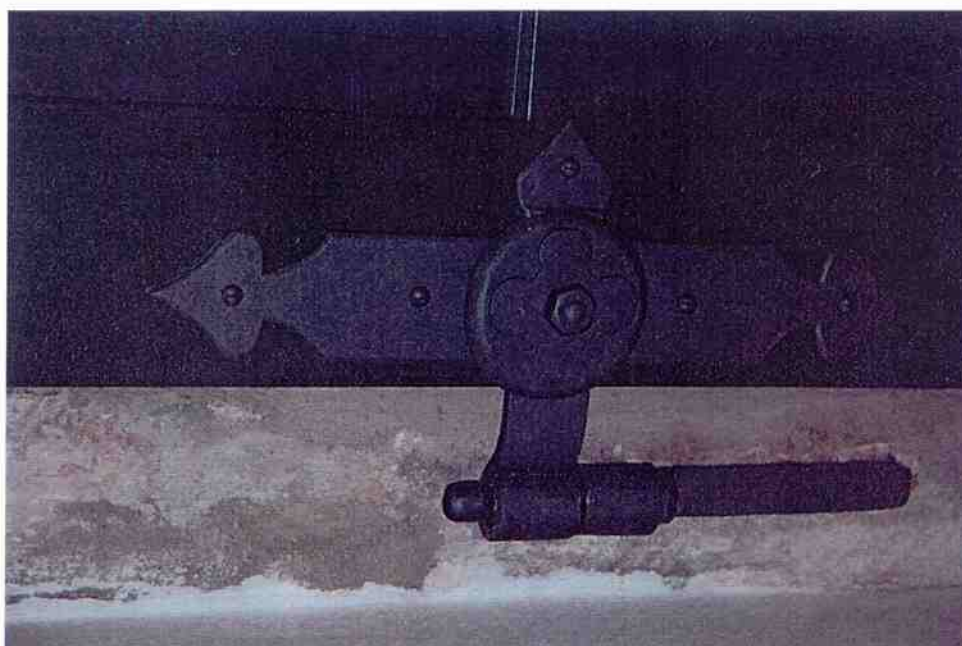
2.26. Dvoukřídlé vchodové dveře, Česká ulice č. p. 263, Kutná Hora Levý dolní dveřní závěs. Pohled z vnitřní strany. Stav po ukončení opravy.
